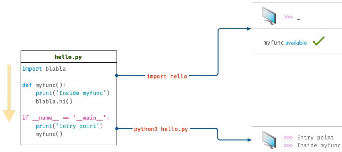
Figura 26: Comportamiento de un programa principal al importarlo o ejecutarlo
