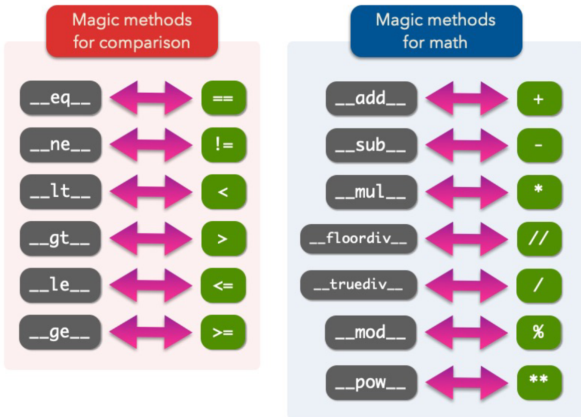
Figura 17: Métodos mágicos para comparaciones y operaciones matemáticas
