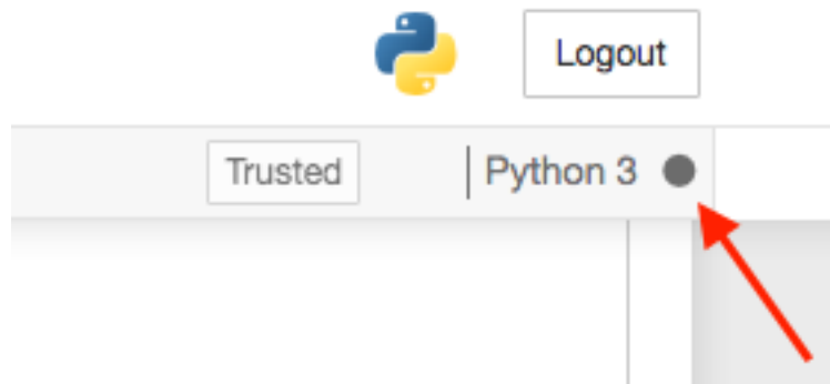
Figura 9: Kernel ocupado
