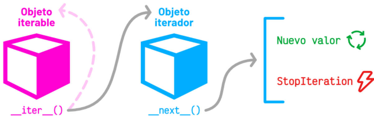
Figura 22: Protocolo de iteración
