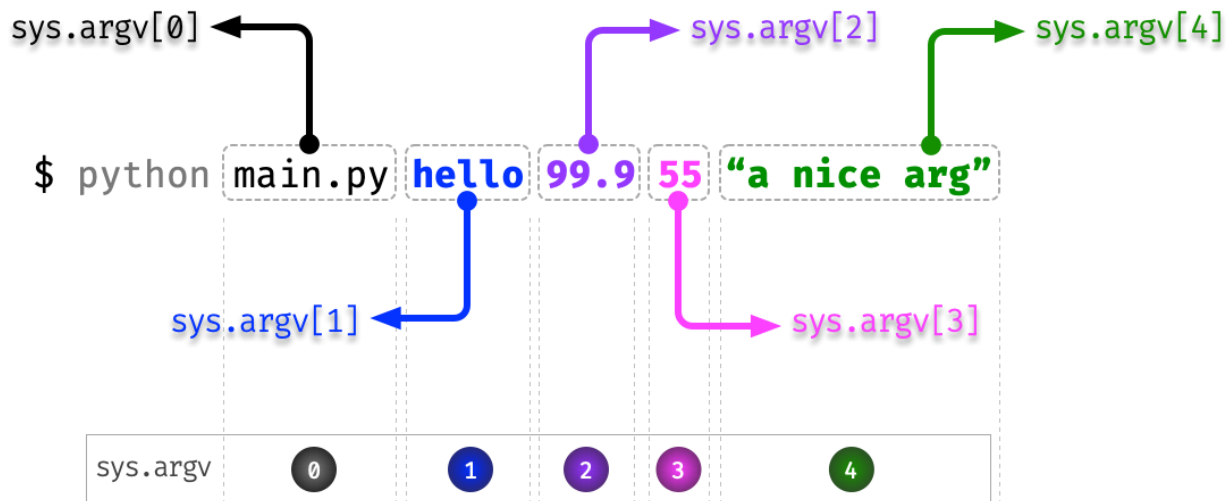
Figura 5: Acceso a parámetros en línea de comandos
