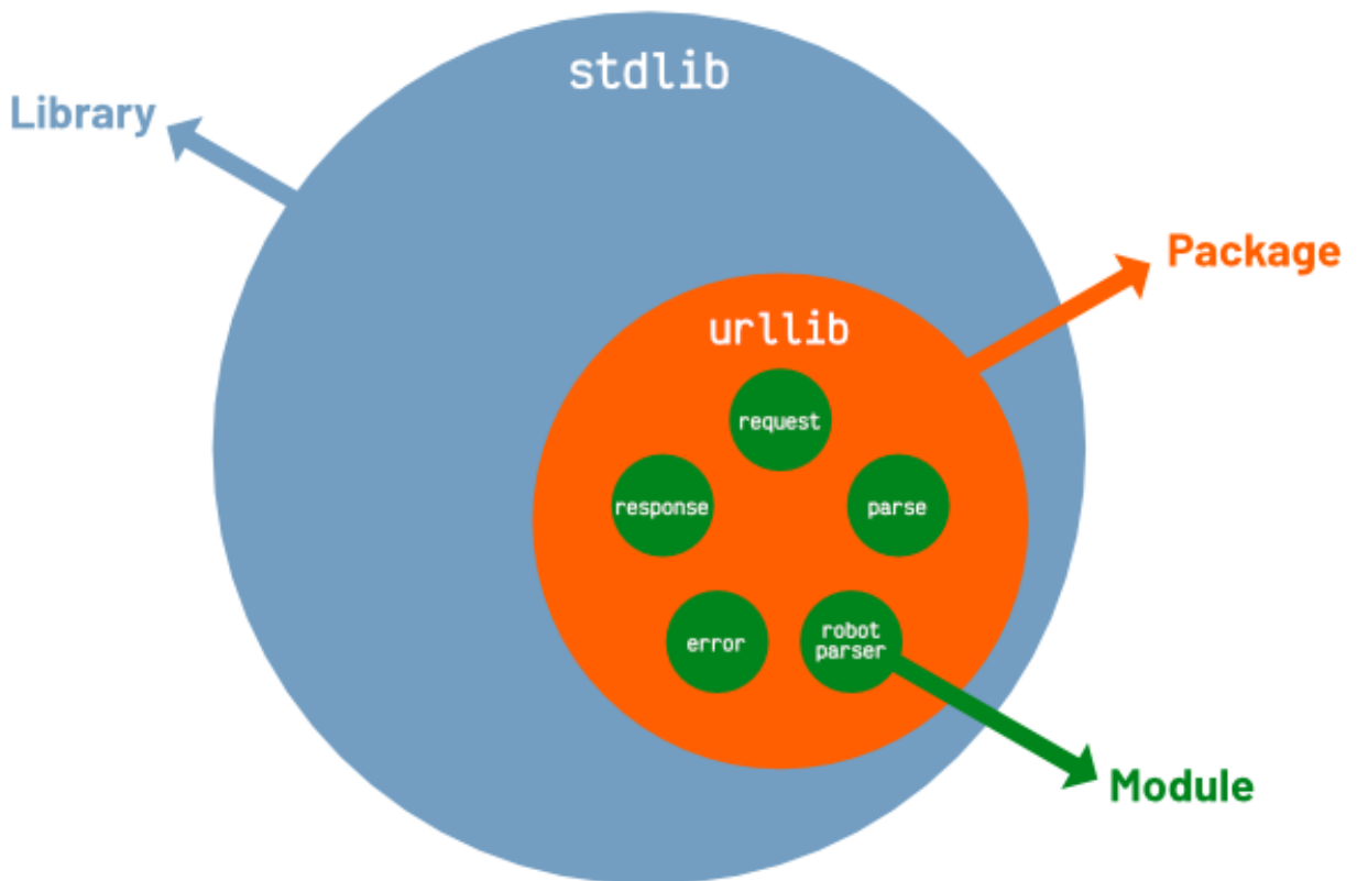
Figura 24: Ejemplo de paquete y módulos en la librería estándar
